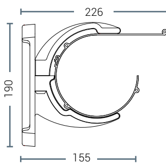
INGOMBRO
