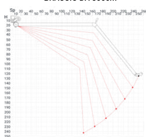
BRACCIO DA 300cm
