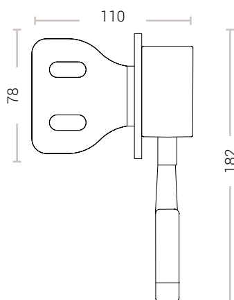
STAFFA A PARETE
