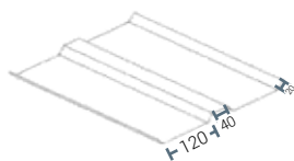
GRONDAIA CENTRALE
