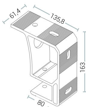
STAFFA UNIVERSALE
