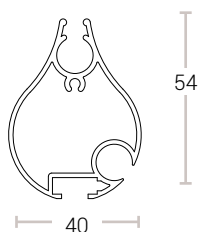
TERMINALE
