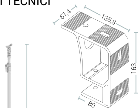
STAFFA UNIVERSALE
