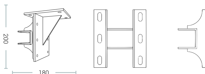
STAFFA UNIVERSALE
