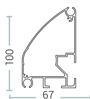
TERMINALE
