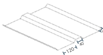
GRONDAIA CENTRALE
