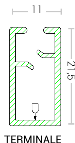
TERMINALE
