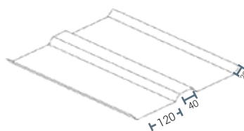
GRONDAIA CENTRALE
