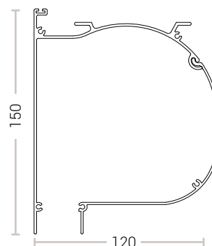
CASSONETTO
