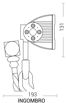
INGOMBRO
