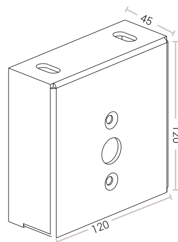
STAFFA
