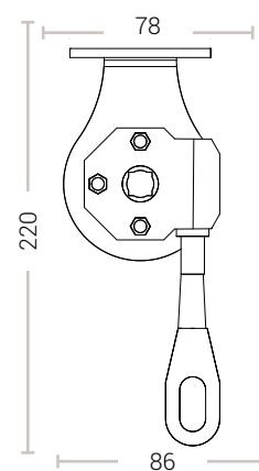
STAFFA A SOFFITTO
