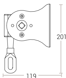
MONTAGGIO A PARETE
