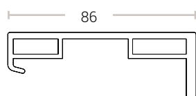
STAFFA A SOFFITTO VISTA LATERALE
