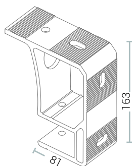
STAFFA UNIVERSALE
