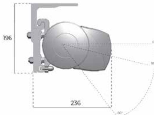
INGOMBRO MONTAGGIO A SOFFITTO
