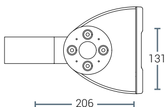
STAFFA VISTA LATERALE
