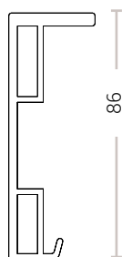
STAFFA A SOFFITTO VISTA LATERALE
