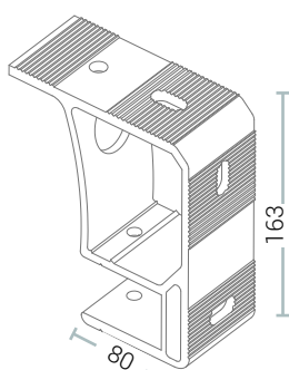
STAFFA UNIVERSALE
