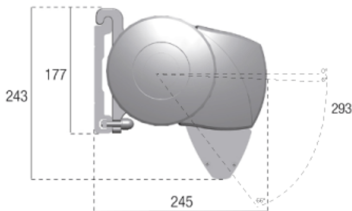
INGOMBRO MONTAGGIO A PARETE
