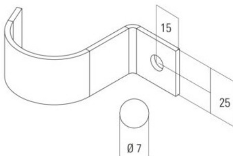
CURVA
