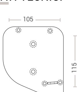
TESTATA CASSONETTO
