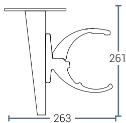
STAFFA A SOFFITTO
