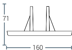
PIEDINO
