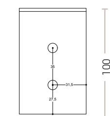
STAFFA A SOFFITTO VISTA LATERALE
