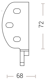
STAFFA VISTA POSTERIORE
