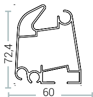
TERMINALE
