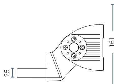
STAFFA SENZA CASSONETTO
