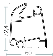
TERMINALE
