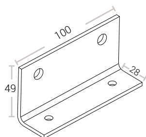
STAFFA INTERNO VANO
