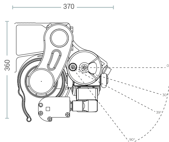
INGOMBRO
