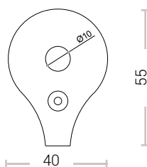
TENDICAVO SNODABILE
