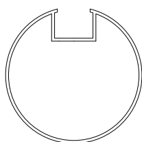
PROFILO
