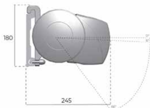
INGOMBRO MONTAGGIO A PARETE
